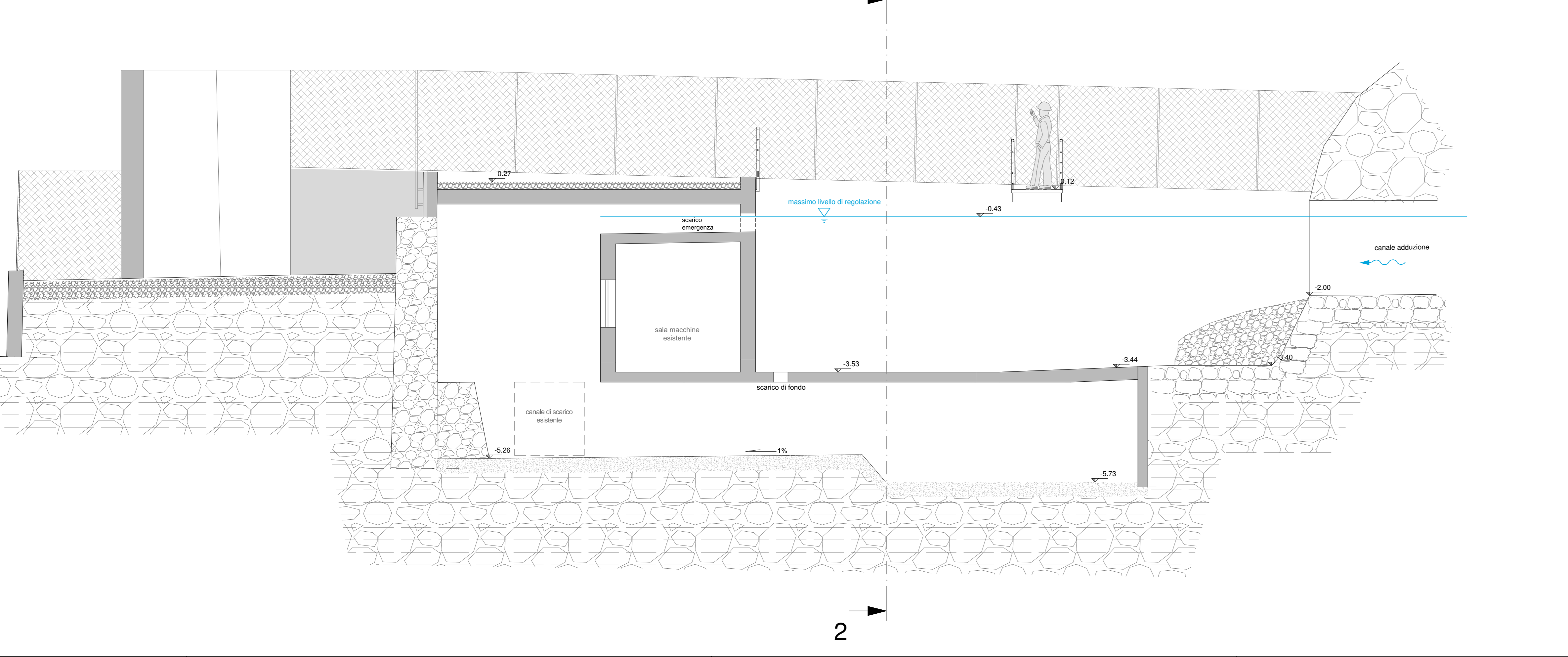
Sezione 1-1 Scala 1:50
