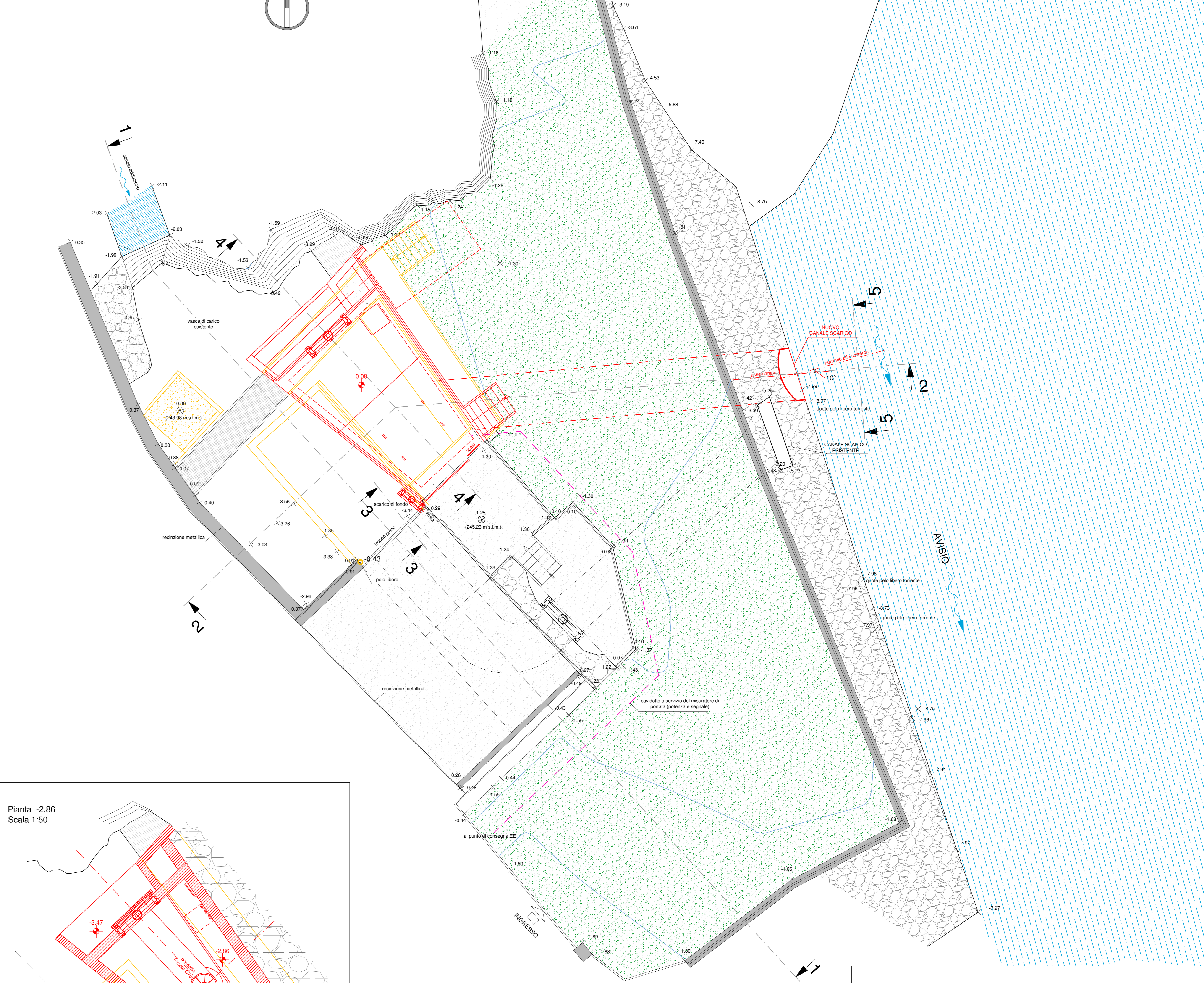
Planimetria Scala 1:50
