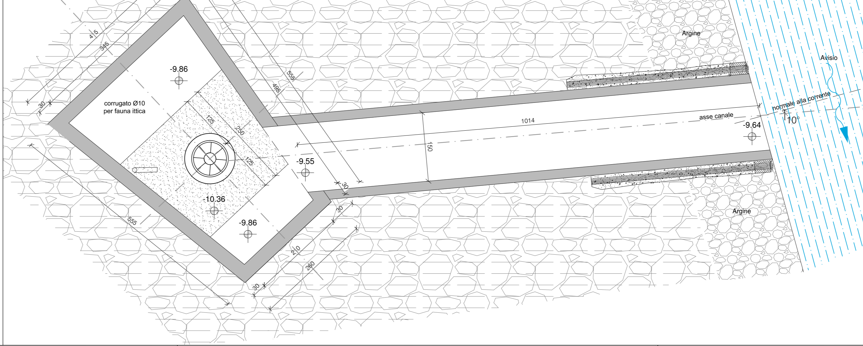
Pianta -9.86/-10.36 Scala 1:50
