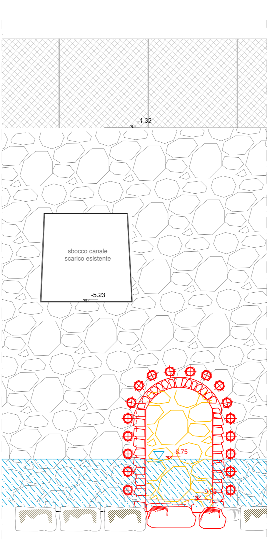
Sezione 5-5 Scala 1:50
