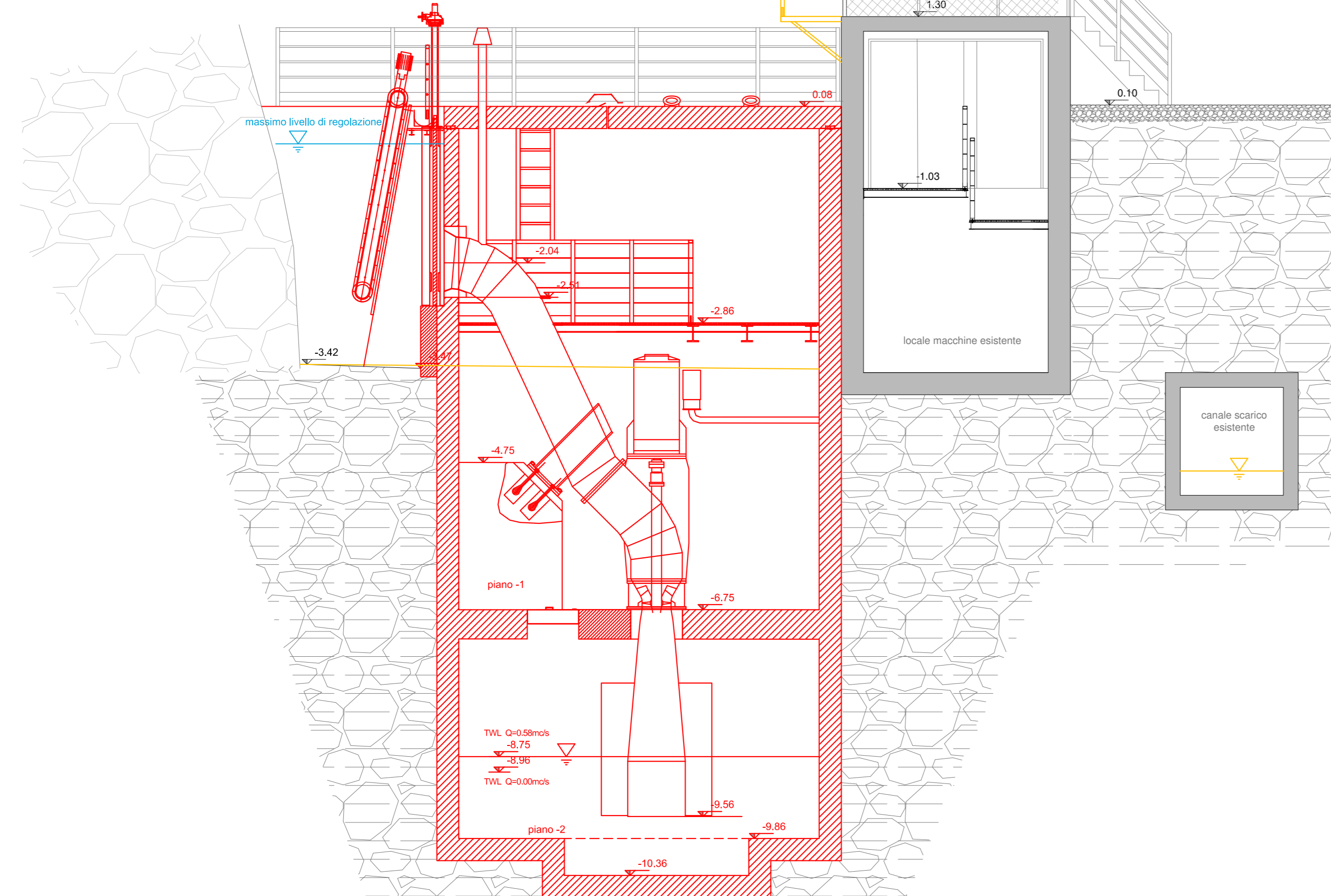
Sezione 4-4 Scala 1:50
