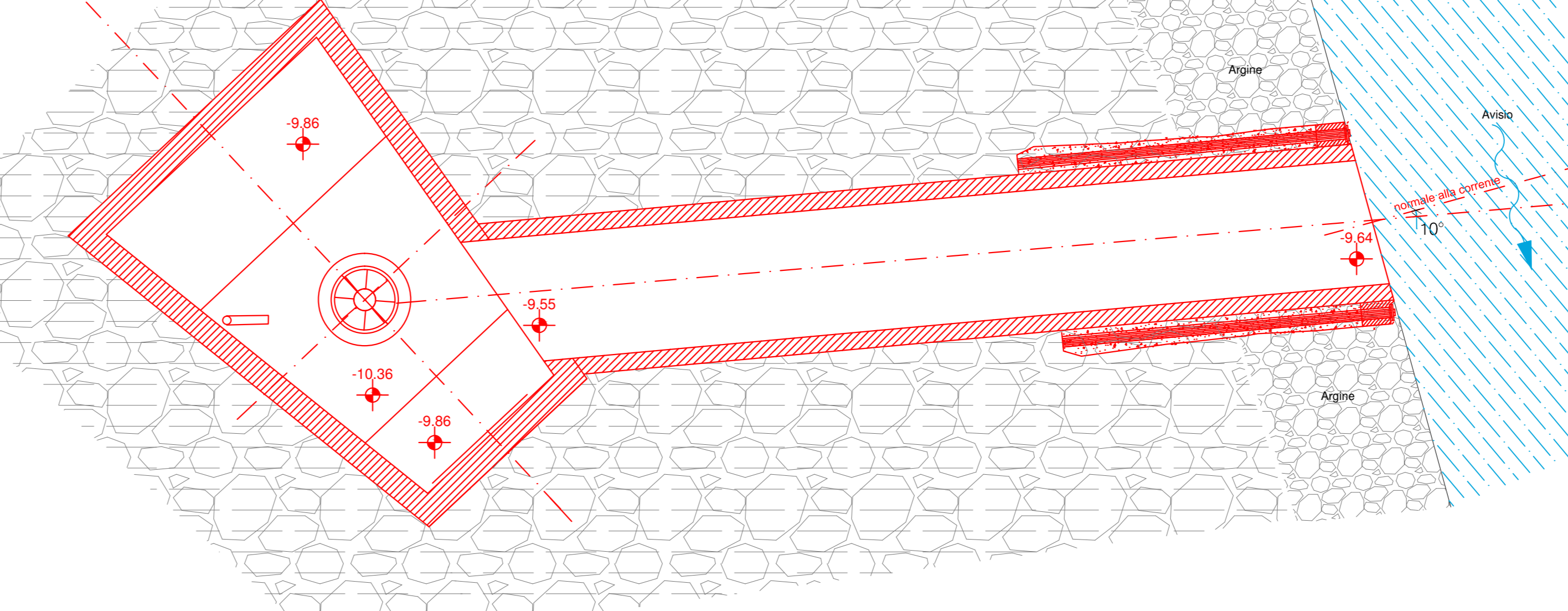
Pianta -9.86/-10.36 Scala 1:50
