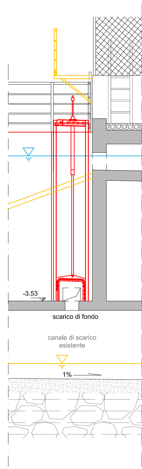
Sezione 3-3 Scala 1:50
