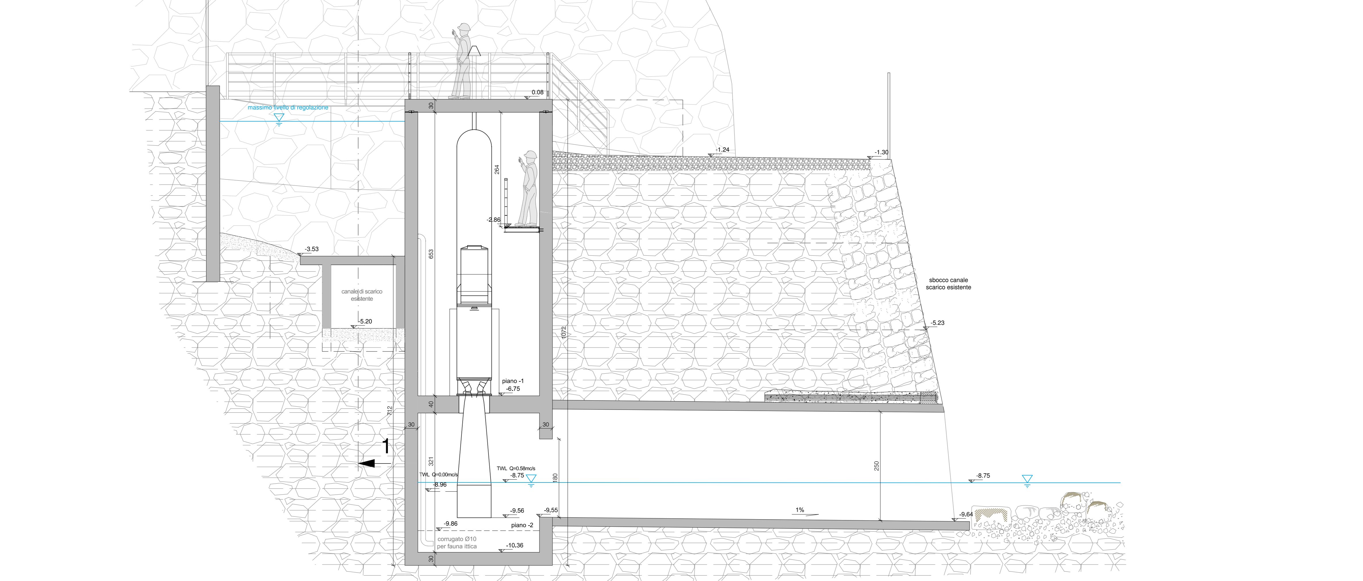
Sezione 1-1 Scala 1:50
