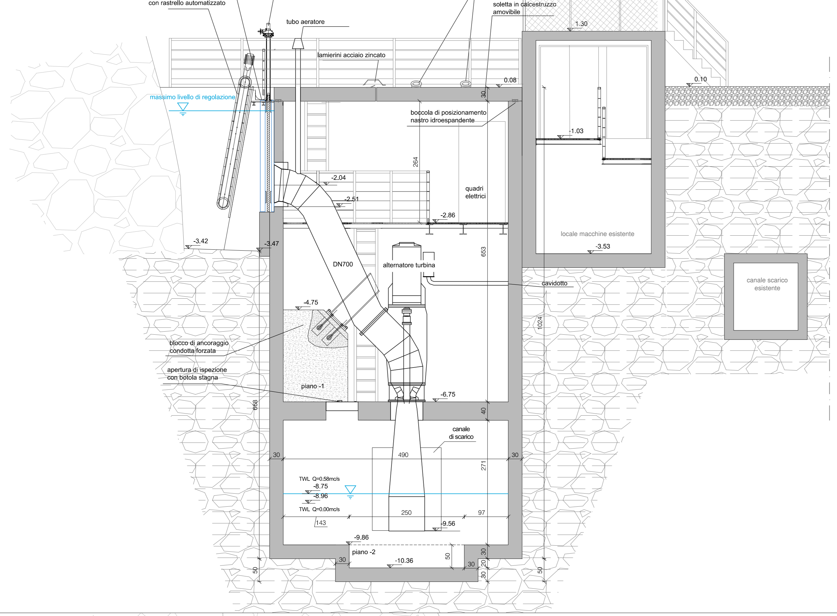
Sezione 4-4 Scala 1:50
