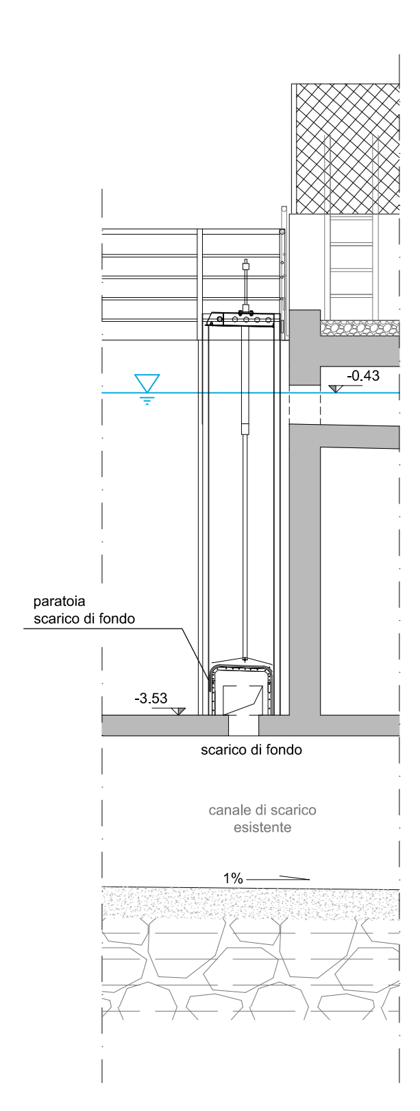
Sezione 3-3 Scala 1:50
