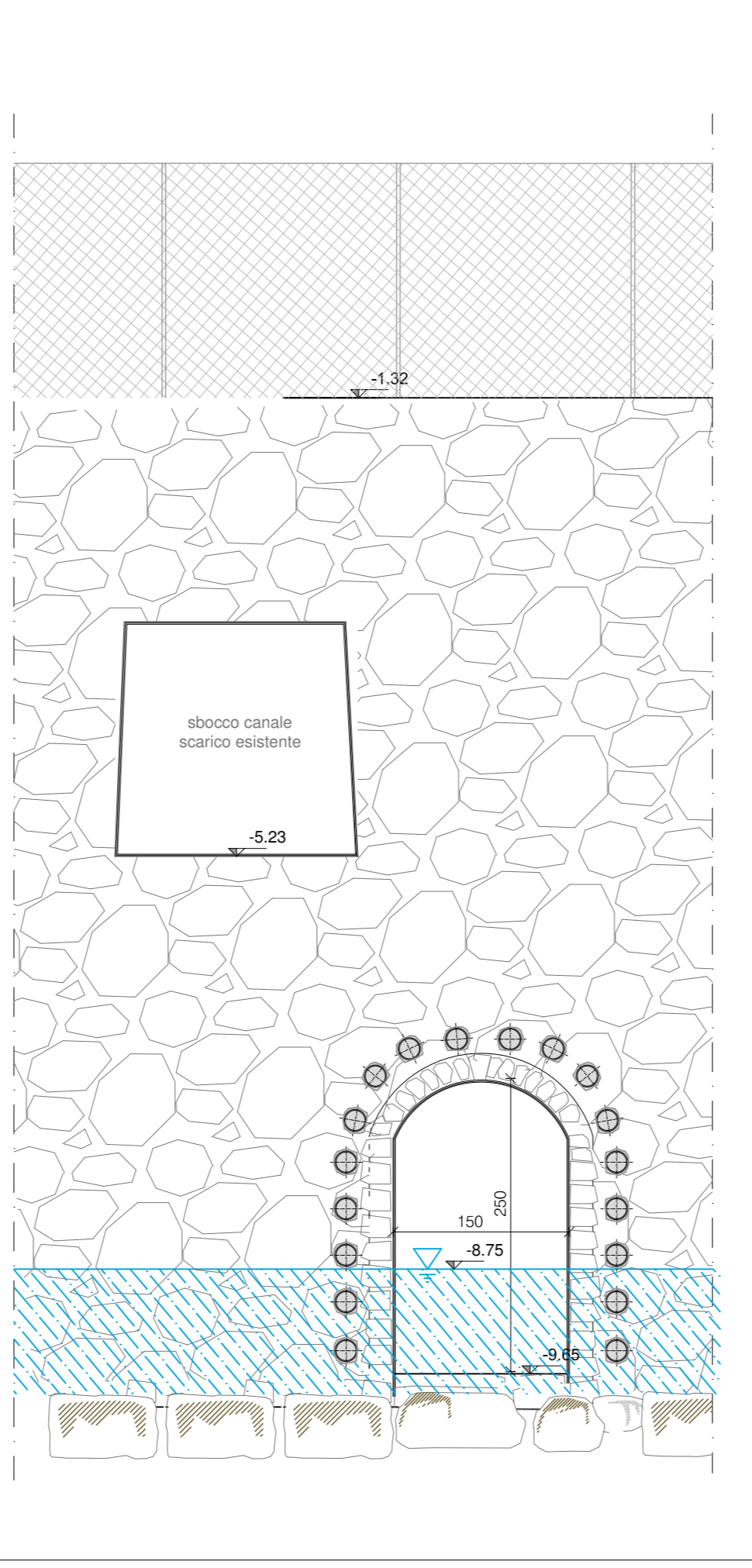
Sezione 5-5 Scala 1:50
